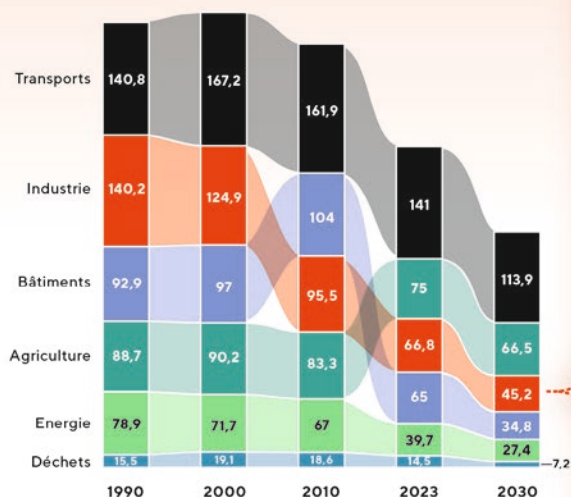
Evolution des émissions par grands secteurs et projection (en millions de tonnes équivalent CO 2 par an)
